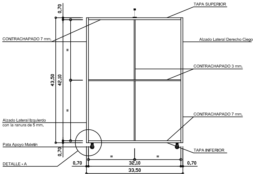
ALZADO FRONTAL
