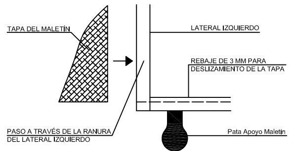
DETALLE - A
